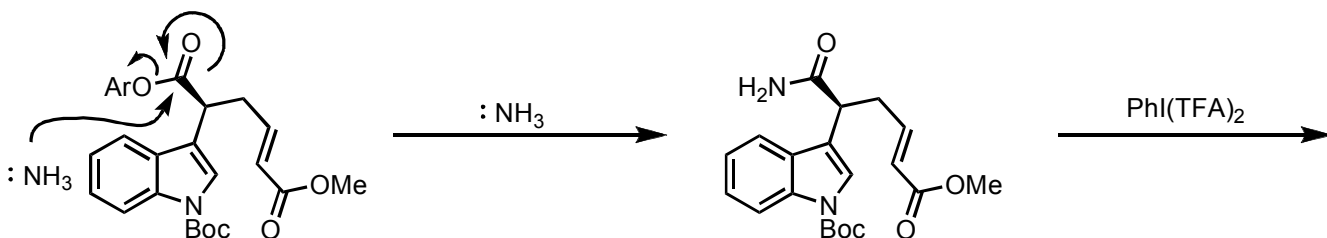
Hofmann rearrangement
