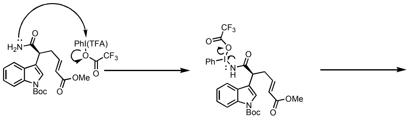
Hofmann rearrangement
