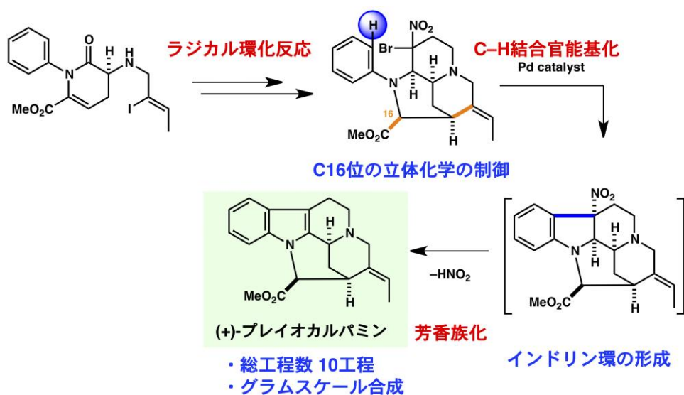
図 2. (+)-プレイオカルパミンの不斉全合成の概略図。
