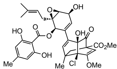
Chloropupukeananin
