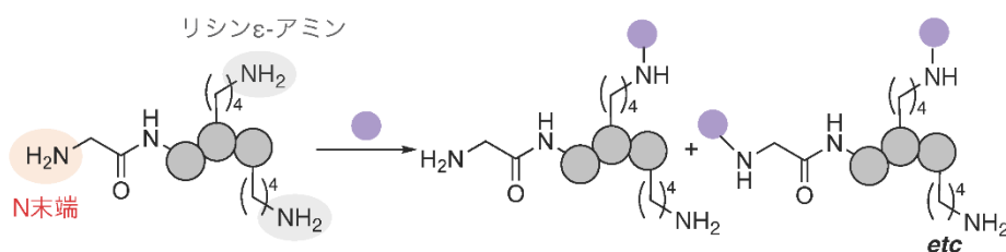
図1. ペプチド修飾の課題：反応点が多く均一な変換は困難
