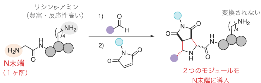
図2. 本研究：N末端のみに2つのモジュールを導入する手法
