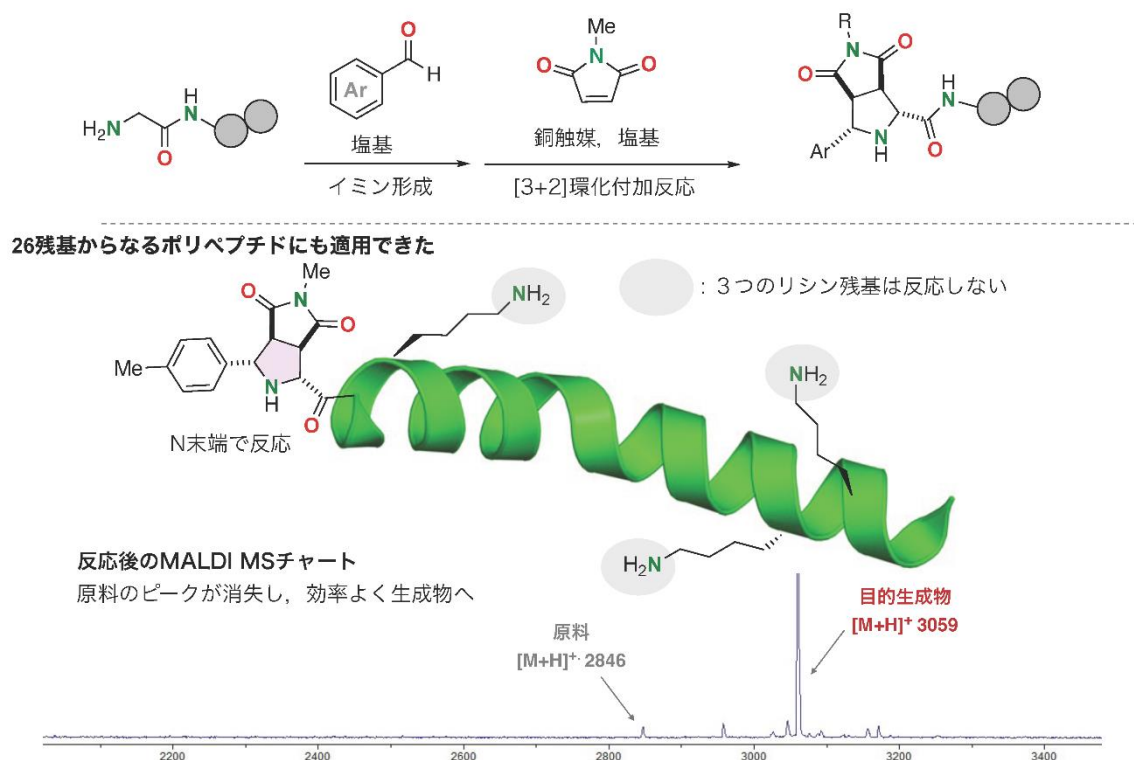
図 4. 様々なアミノ酸残基を持つポリペプチドへの利用
