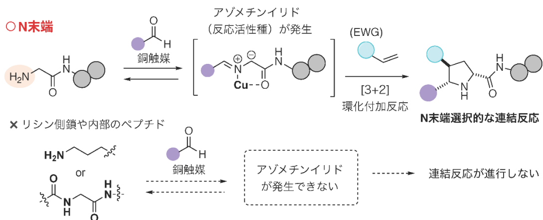
図 3. N 末端選択性の原理
