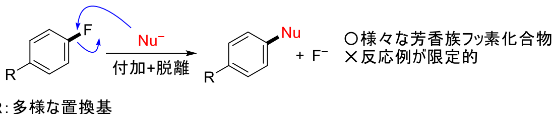
図 1. 芳香族求核置換( S_NAr )の反応形式。 CS_NAr は古典的な S_NAr と異なり、電子求引基だけでなく多様な置換基を有する芳香族フッ化化合物と反応できることが知られていた。一方で、反応例が散発的に見つかるだけで、限定的だった。
