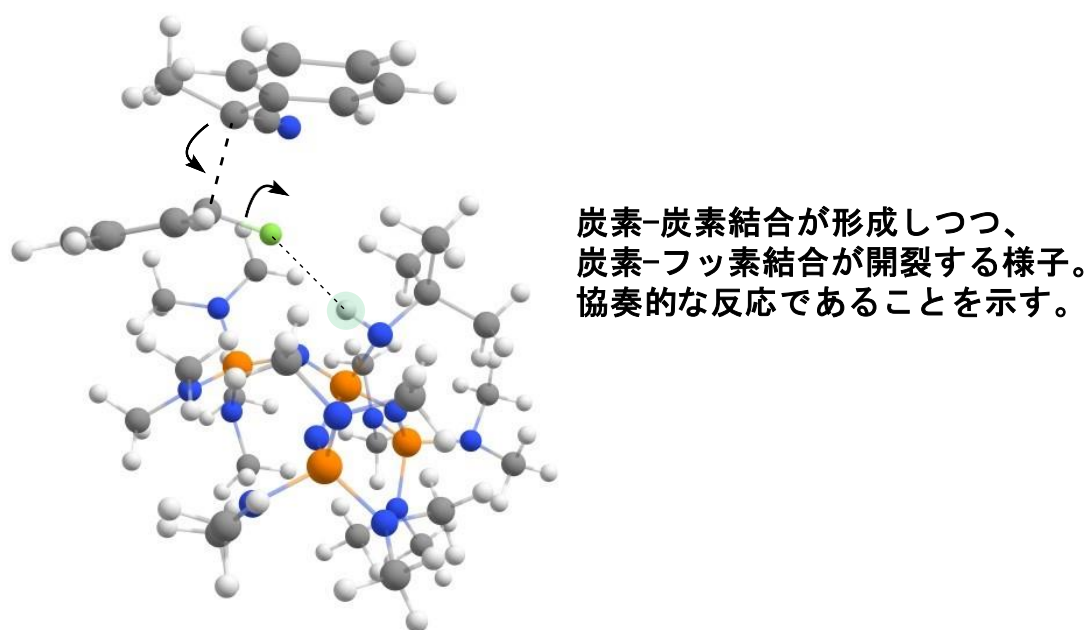
図 3. 計算科学で得られた \text{CS}_\text{N}\text{Ar} 反応の遷移状態 (注 14) 。上から近づいてきた求核剤 ( \text{Nu}^- ) 中の炭素原子 (灰色の丸) とフルオロアレーン ( \text{Ph-F} ) 中の炭素原子との間に炭素-炭素結合 (図中では破線で表示) が形成される。それと同時に \text{Ph-F} 中の炭素原子とフッ素原子 (黄緑色の丸) の間の炭素-フッ素結合が開裂する。 t\text{-Bu-P4} 触媒が存在することで、このような協奏的な反応が起こる。
