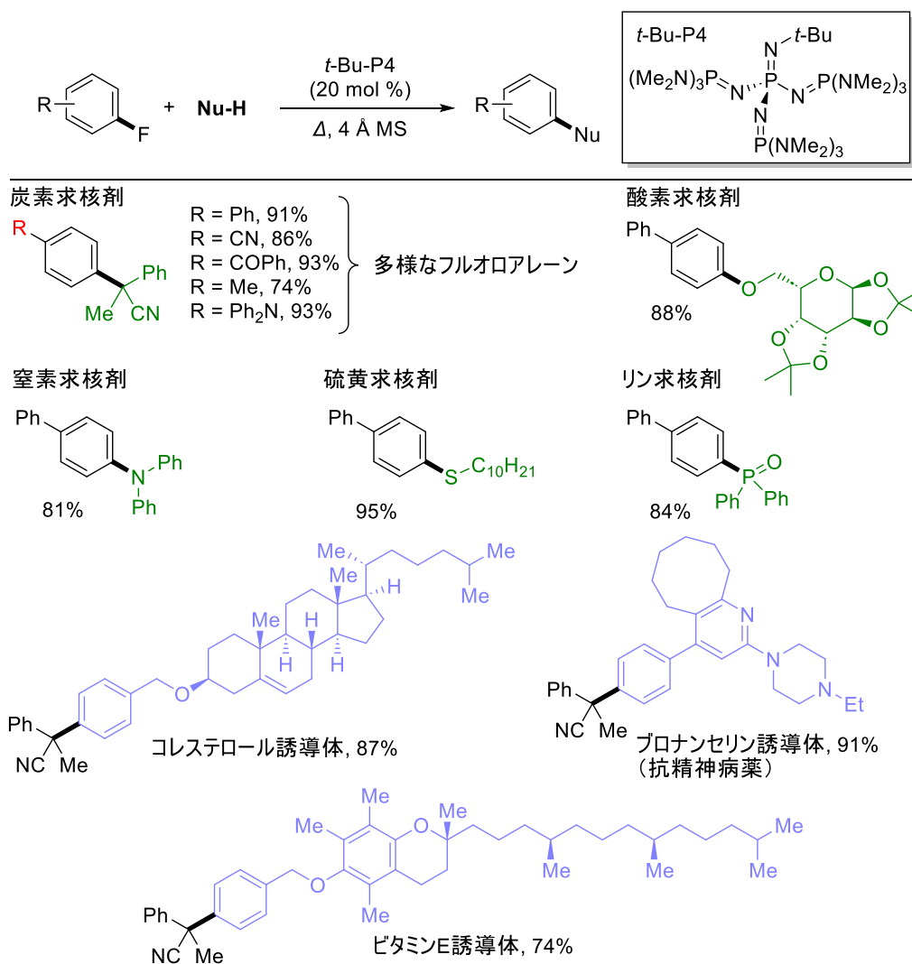
図 2. 今回開発した t -Bu-P4 触媒を用いた \text{CS}_\text{N}\text{Ar} 反応。多様なフルオロアレーンや求核剤が利用できる(一部抜粋)。
