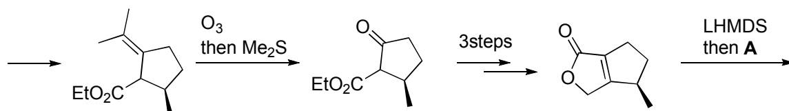
Ozonolysis
